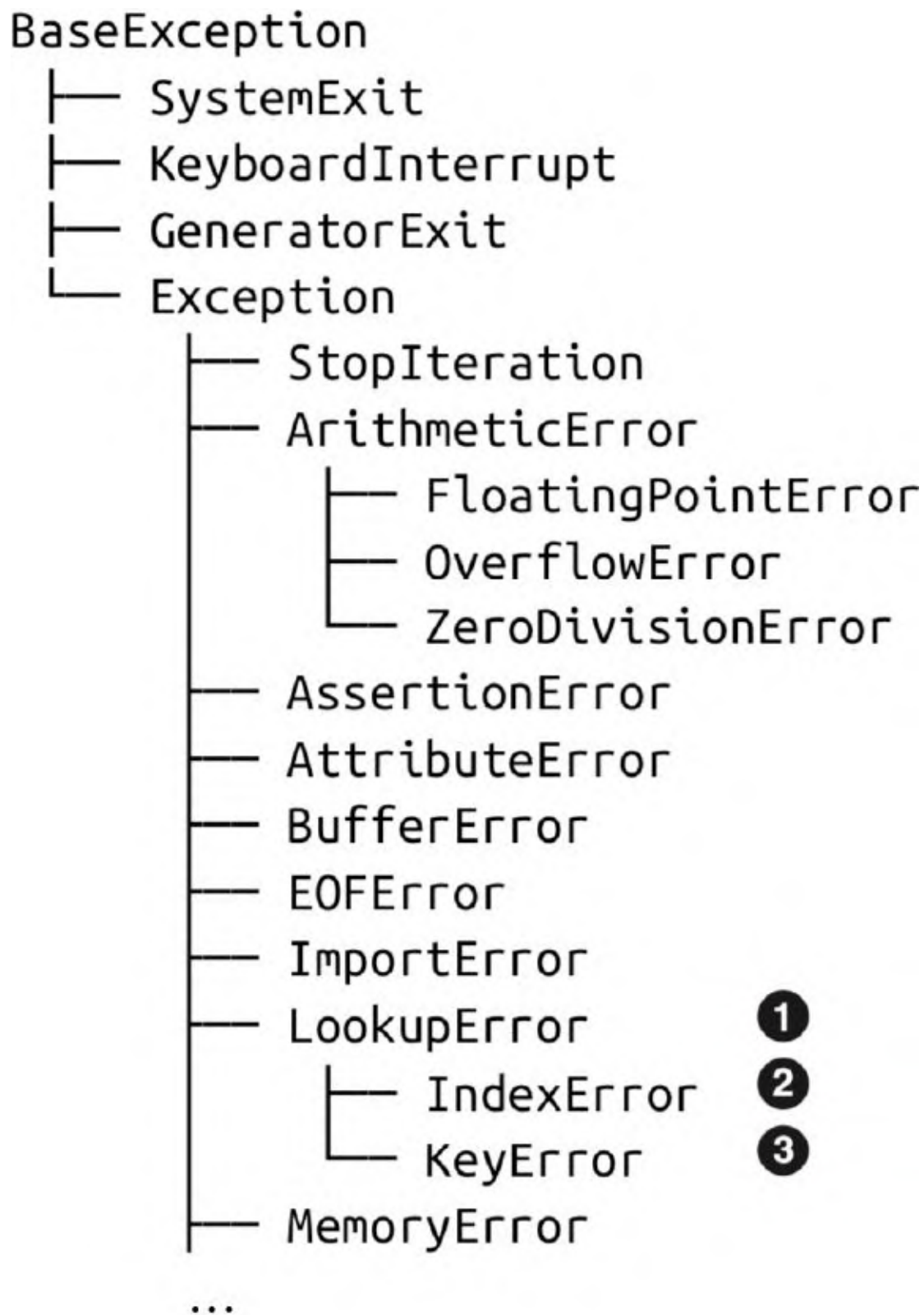
图 13-6: Exception 类的部分层次结构 10
