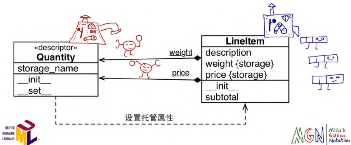
图 23-2: 带有 MGN (Mills & Gizmos Notation, 机器和小怪兽图示法) 注解的 UML 类图: 类是机器, 用于生产小怪兽 (实例)。
