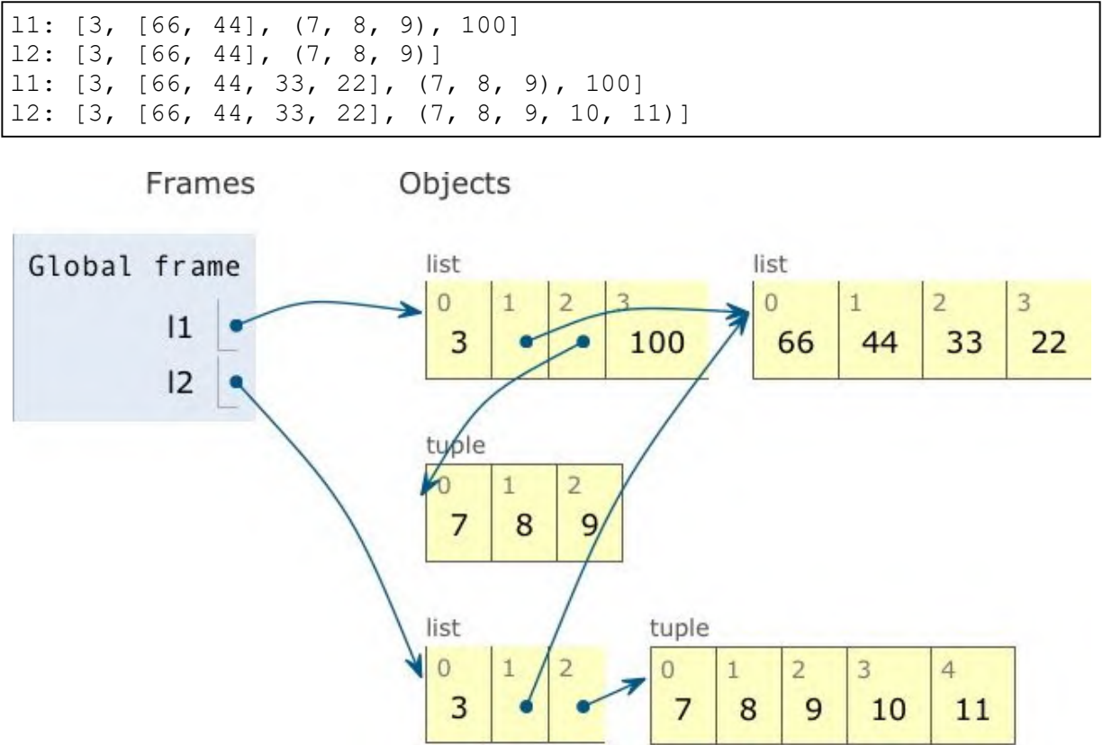
图 6-4: l1 和 l2 的最终状态：二者依然引用同一个列表对象，现在列表的值是 [66, 44, 33, 22] ，不过 l2[2] += (10, 11) 操作创建一个新元组，内容是 (7, 8, 9, 10, 11) ，它与 l1[2] 引用的元组 (7, 8, 9) 无关（截图由 Python Tutor 网站生成）
