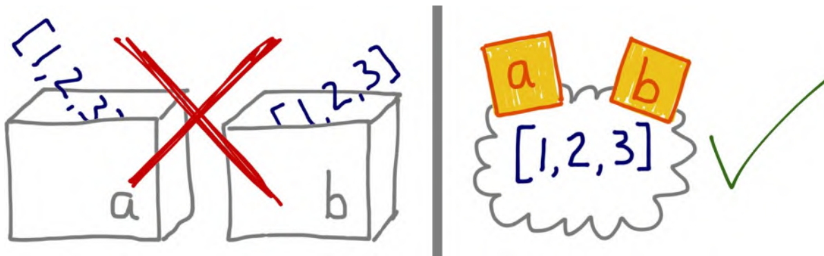
图 6-1：把变量想象为盒子，无法解释 Python 中的赋值。应该把变量视作便利贴，这样就好解释示例 6-1 中的行为了
