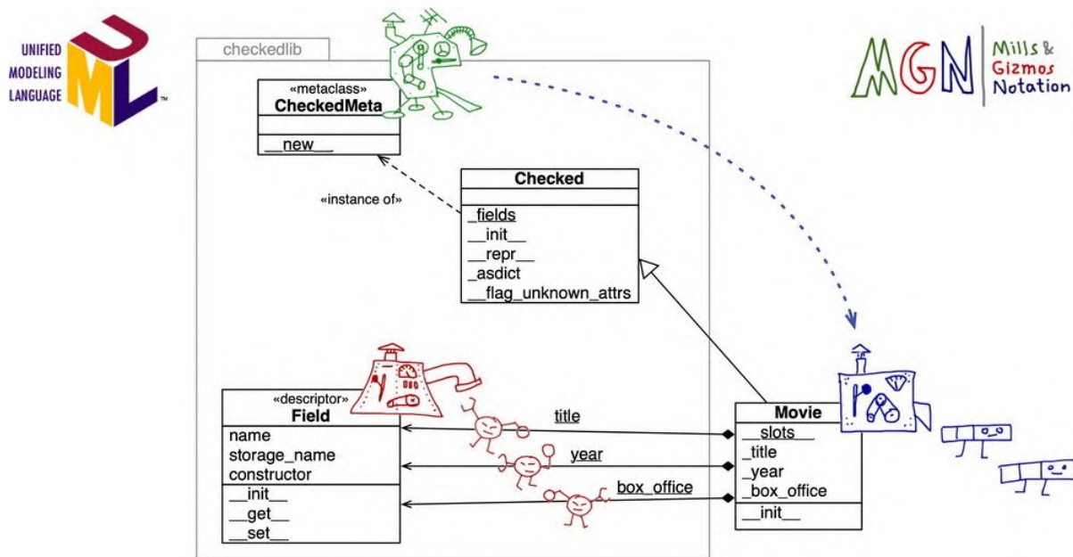
图 24-4：使用 MGN 注解的 UML 类图。 CheckedMeta 元机器构建 Movie 机器。 Field 机器构建描述符 title 、 year 和 box_office ——这些都是 Movie 的类属性。各个实例的字段数据存储在 Movie 的实例属性 _title 、 _year 和 _box_office 中。注意 checkedlib 包的边界。 Movie 的开发人员无须熟谙 checkedlib.py 的内部机制
