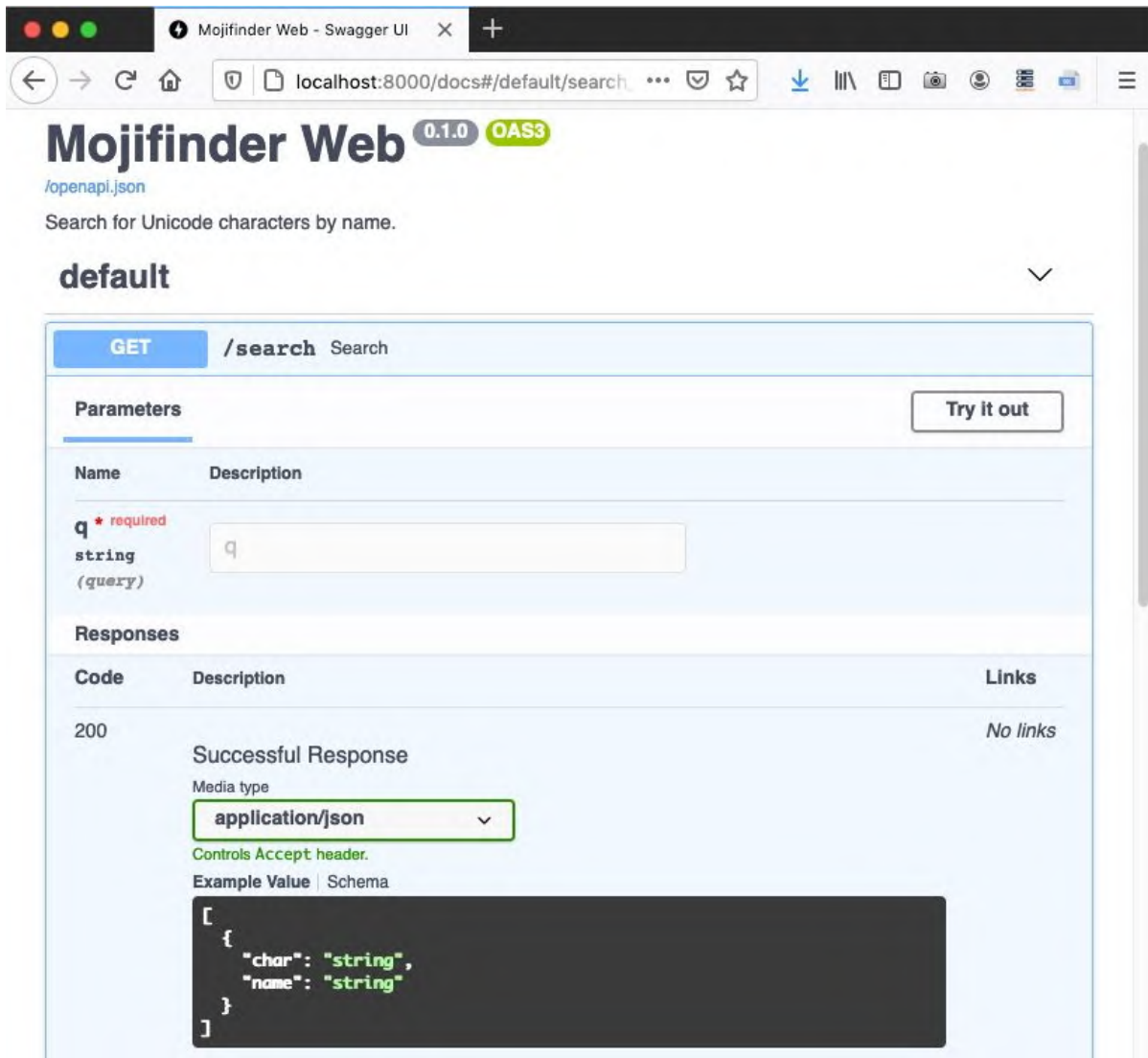
图 21-4: 为 /search 端点自动生成的 OpenAPI 模式
