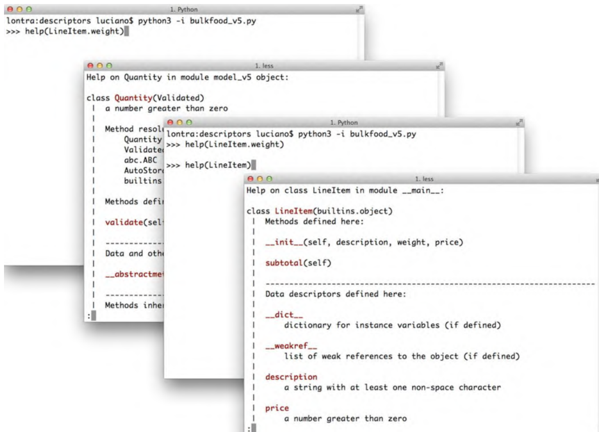
图 23-4: 在 Python 控制台中执行 help(LineItem.weight) 命令和 help(LineItem) 命令时的界面截图
