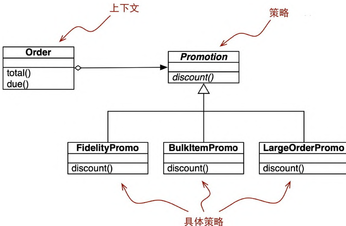
图 10-1：使用策略设计模式处理订单折扣的 UML 类图
